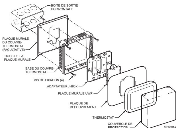
Fig. 2. Montage de la plaque murale du couvre-thermostat, de la base du couvre-thermostat et du thermostat sur une boîte de jonction.
