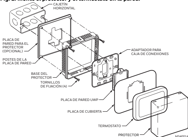
Fig. 2. Monte la placa de pared para el protector con la base del protector y el termostato en la caja de conexiones.
